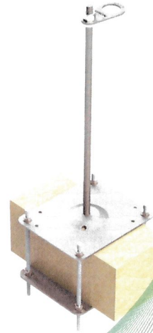
Bild 6: Anschlageinrichtung, Typ: SAFEX-ESE MULTI mit Konterplatte montiert auf Holz
