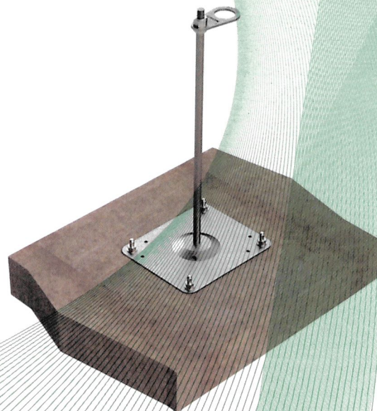
Bild 2: Anschlagereinrichtung, Typ: SAFEX-ESE MULTI montiert auf Beton
