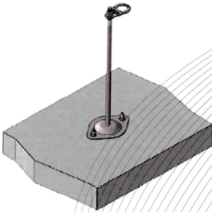
Bild 7: Anschlageinrichtung, Typ: SAFEX-ESE MULTI 2- Loch montiert auf Beton
