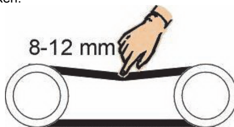
Abb. Keilriemenspannung
